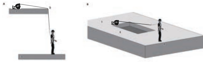
Figure 7 - Utilisation incorrecte du DAR de bord d'attaque A Ne pas soumettre la ligne de vie du câble à un bord d'attaque ou à un bord tranchant pendant une utilisation normale. B Ne pas ancrer le DAR sur le côté opposé du trou existant ou de l'ouverture du plancher à partir du lieu de travail.
