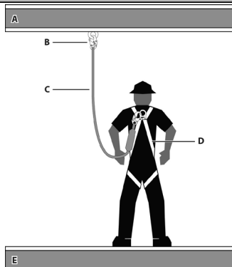
Figure 7 - Blocage des chutes (PFAS)
