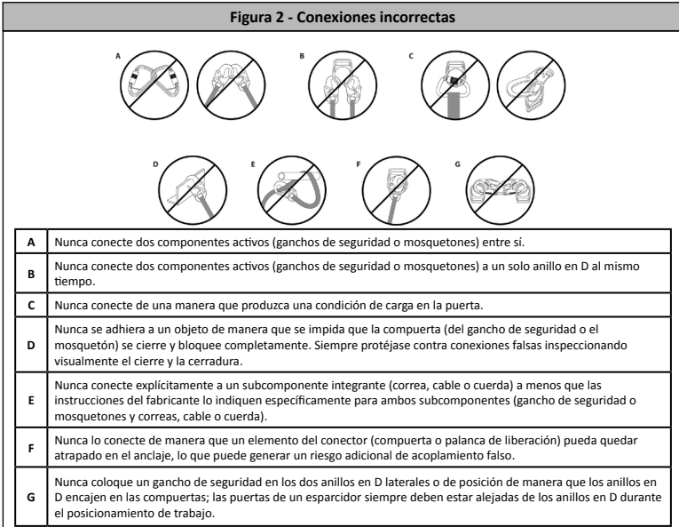
Figura 2 - Conexiones incorrectas
