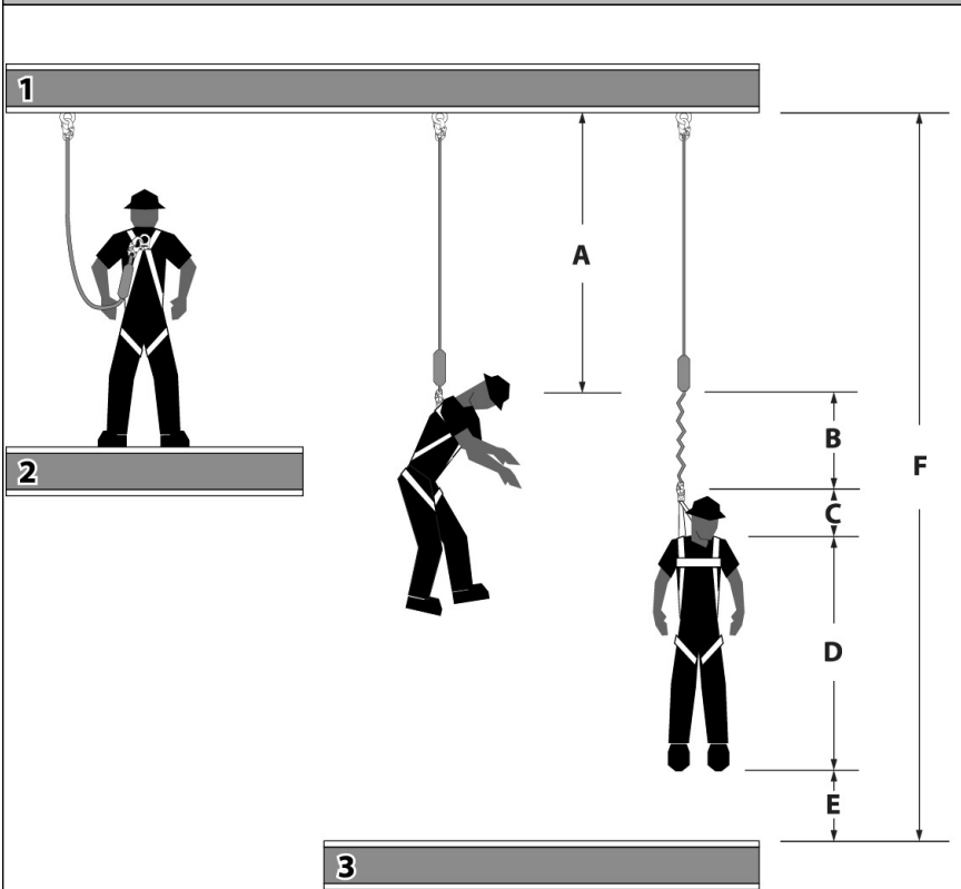
Figure 1 - Dégagement minimal requis en cas de chute : Cordon amortisseur d'énergie de 6 pieds. Mesuré à partir du point d'ancrage supérieur
